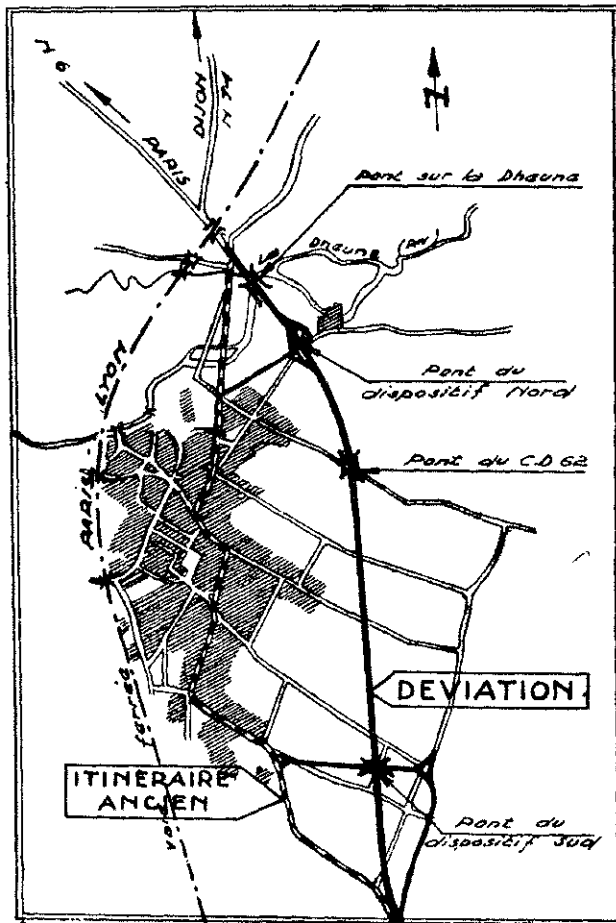
Plan d'ensemble de la déviation
